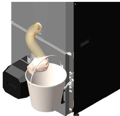
Rysunek 29 - Test podajnika
