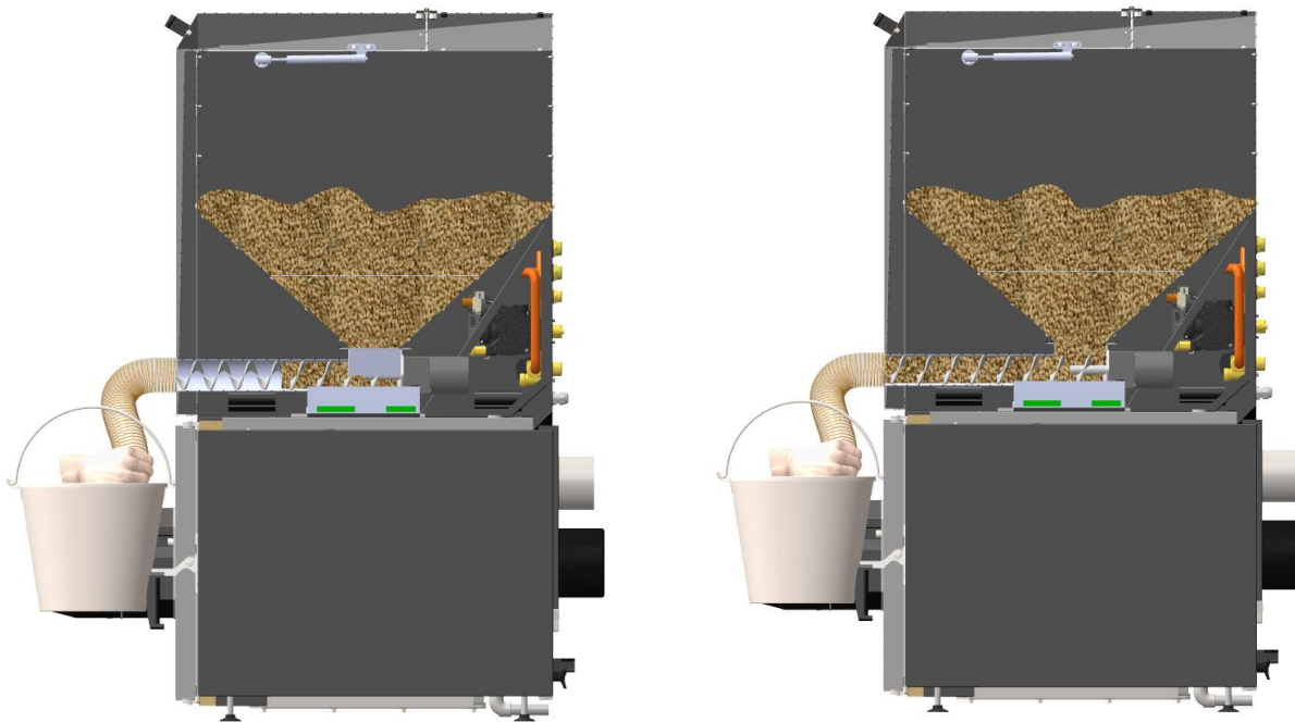
Rysunek 28 – Napełnianie podajnika
