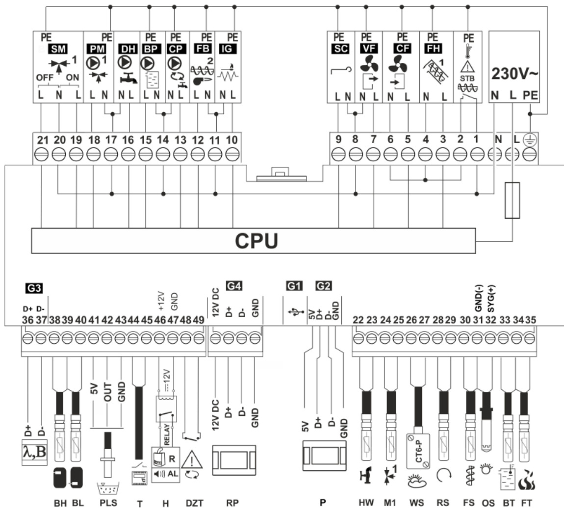
Rysunek 25 - Schemat połączeń elektrycznych regulatora: \lambda – moduł sondy Lambda, B – moduł do obsługi dodatkowych obiegów grzewczych, BH – czujnik temperatury bufora górnego typu CT4, BL – czujnik temperatury bufora dolnego typu CT4, PLS – czujnik poziomu paliwa, T – termostat pokojowy (zwierno-rozwierny), H – wyjście napięciowe do sterowania kotłem rezerwowym R lub do sygnalizacji alarmów AL , RELAY – przekaźnik 12VDC, DZT – czujnik otwarcia drzwi kotła, RP – panel pokojowy ecoSTER TOUCH z funkcją termostatu pokojowego, P – panel sterujący, HW – czujnik temperatury CWU typu CT4, M1 – czujnik temperatury obiegu regulowanego (mieszacza 1) typu CT4, WS – pogodowy czujnik temperatury typu CT6-P, RS – czujnik temperatury wody powracającej do kotła typu CT4, FS – czujnik temperatury podajnika typu CT4, OS – optyczny czujnik jasności płomienia, BT – czujnik temperatury kotła typu CT4, FT – czujnik temperatury spalin typu CT2S, L N PE – zasilanie sieciowe 230V~, CPU – sterowanie, STB – wejście do ogranicznika temperatury bezpieczeństwa, FH – podajnik główny, CF – wentylator nadmuchiwy palnika, VF – wentylator wyciągowy, SC – silnik obrotowy czyszczenia palnika, IG – zapalarka, FB – podajnik palnika, CP – pompa cyrkulacji CWU, BP – pompa kotła, DH – pompa CWU, PM – pompa mieszacza 1, SM – siłownik mieszacza 1.
