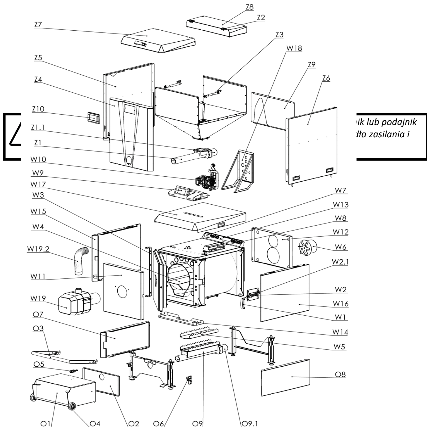
Rysunek 35 – Klasyfikacja części kotła
