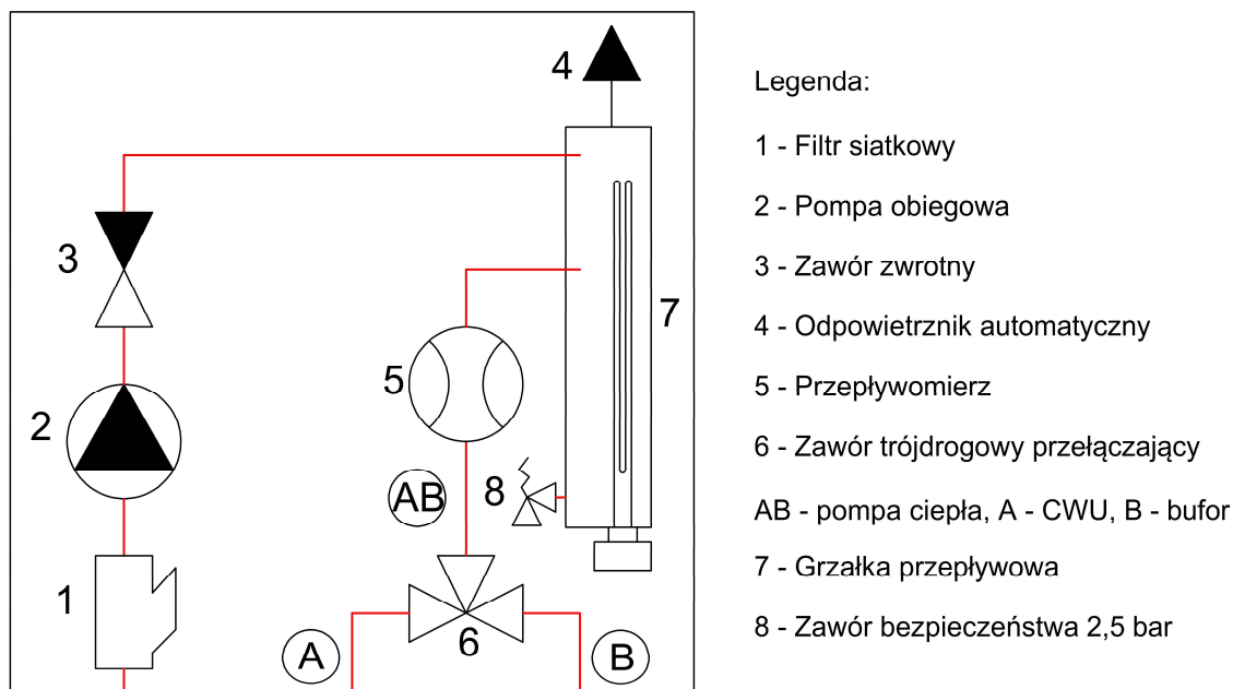
Rysunek 5. Schemat hydrauliczny modułu wewnętrznego HX.
