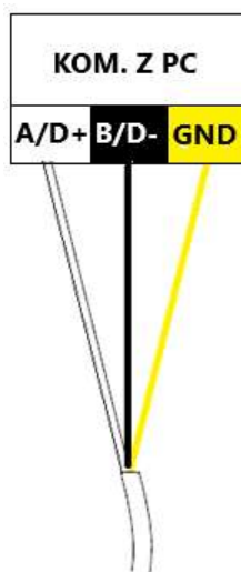
Rysunek 17. Podłączenie przewodu komunikacyjnego.
