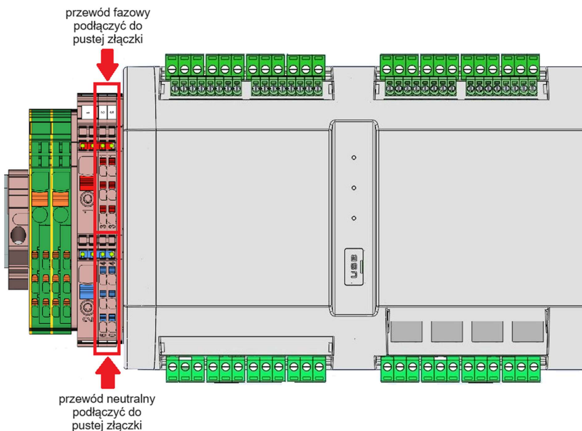
Rysunek 18. Podłączenie zasilania pompy obiegowej.
