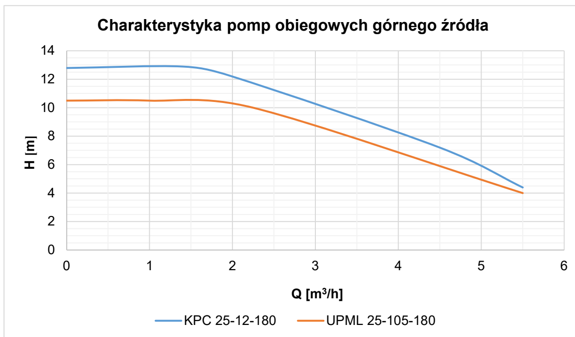
Rysunek 6. Charakterystyka przepływowa pompy obiegowej.
